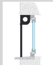
Enroulement intérieur
